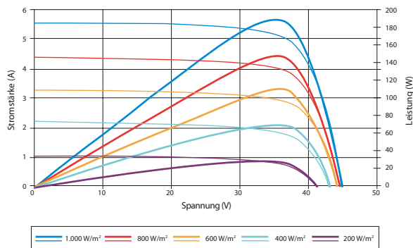
Stromspannungs- & Leistungs-Spannungskennlinie (190S-24)
