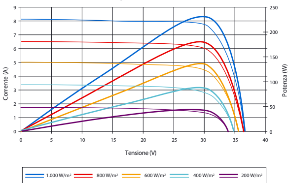
Curve corrente-tensione e potenza-tensione (230-20)
